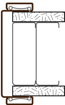
Jamb - No Stop
