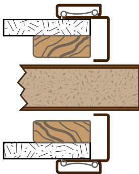
Jamb - Pocket Door Trim
