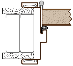
3A Jamb Hinge Side - Kerfed
